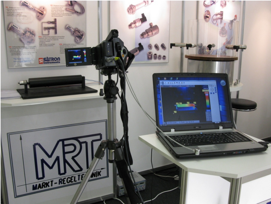
Thermografie des Modell einer beheizten Walze
